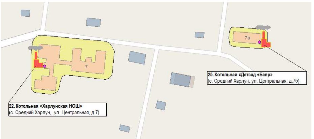
Рис. 2.50. Перспективные зоны действия систем теплоснабжения и централизованных источников тепловой энергии – котельной «Харлунская НОШ» и котельной «Детсад «Баяр»
