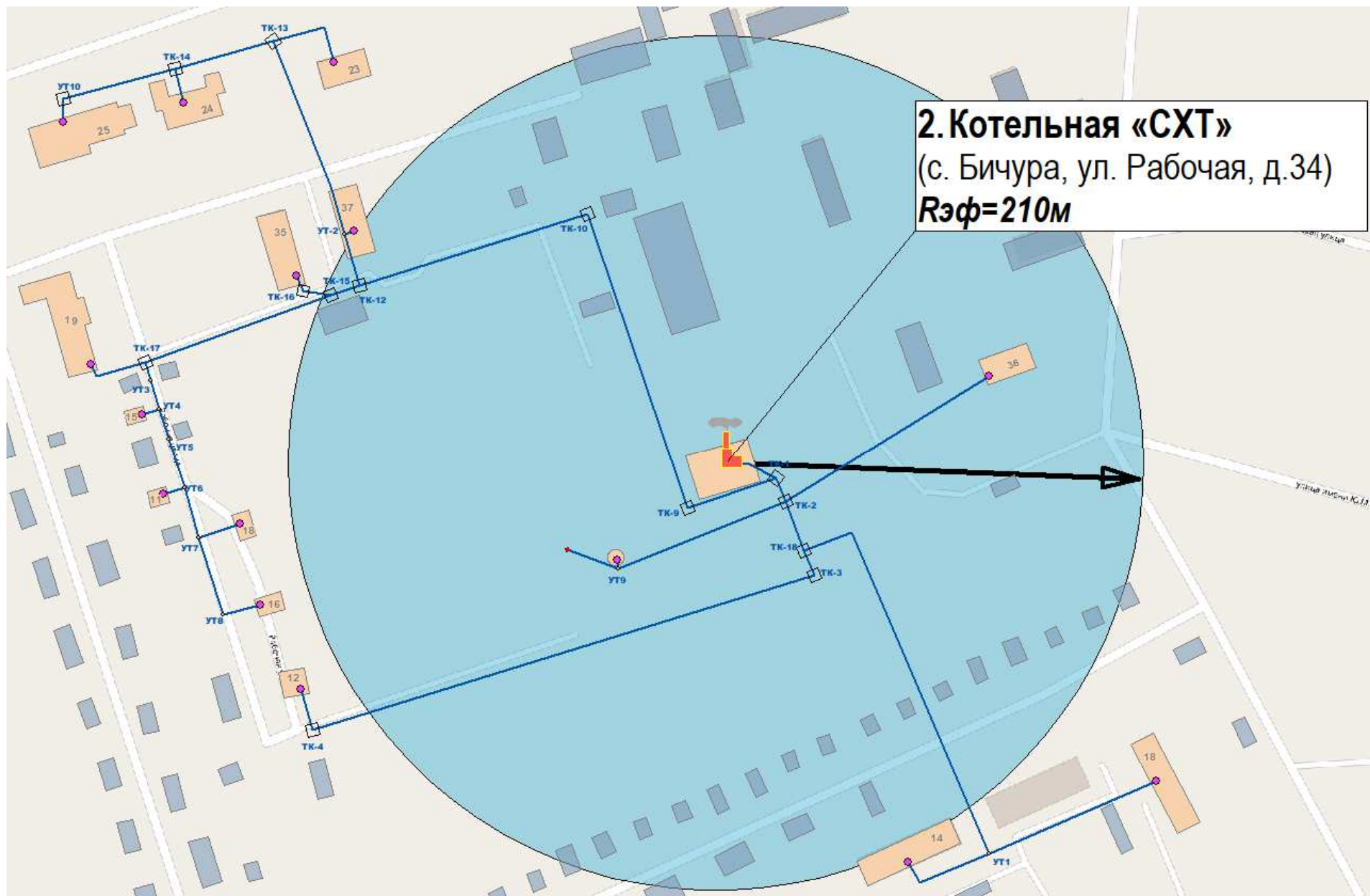
Рис. 2.58. Схема существующего радиуса эффективного теплоснабжения от котельной «СХТ»
