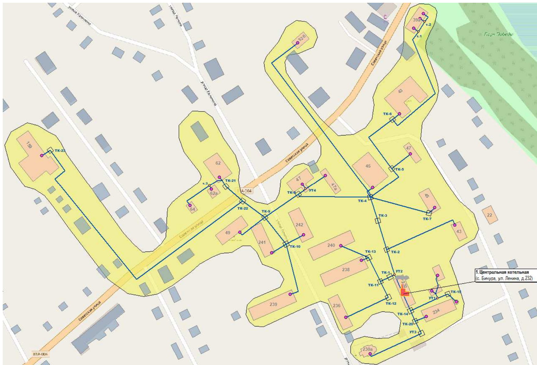
Рис. 2.29. Перспективная зона действия системы теплоснабжения и централизованного источника тепловой энергии – Центральной котельной
