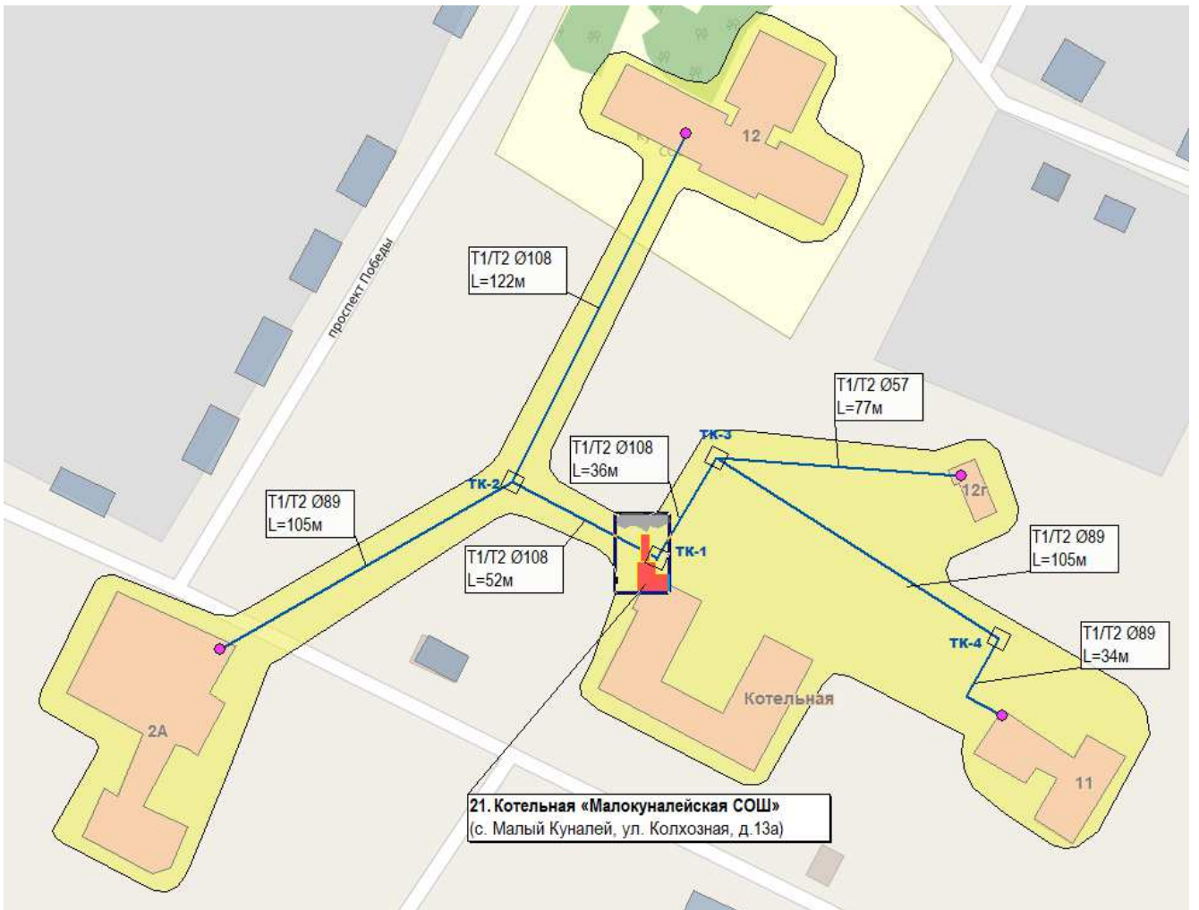
Рис. 2.21. Существующая зона действия системы теплоснабжения и централизованного источника тепловой энергии – котельной «Малокуналейская СОШ»
