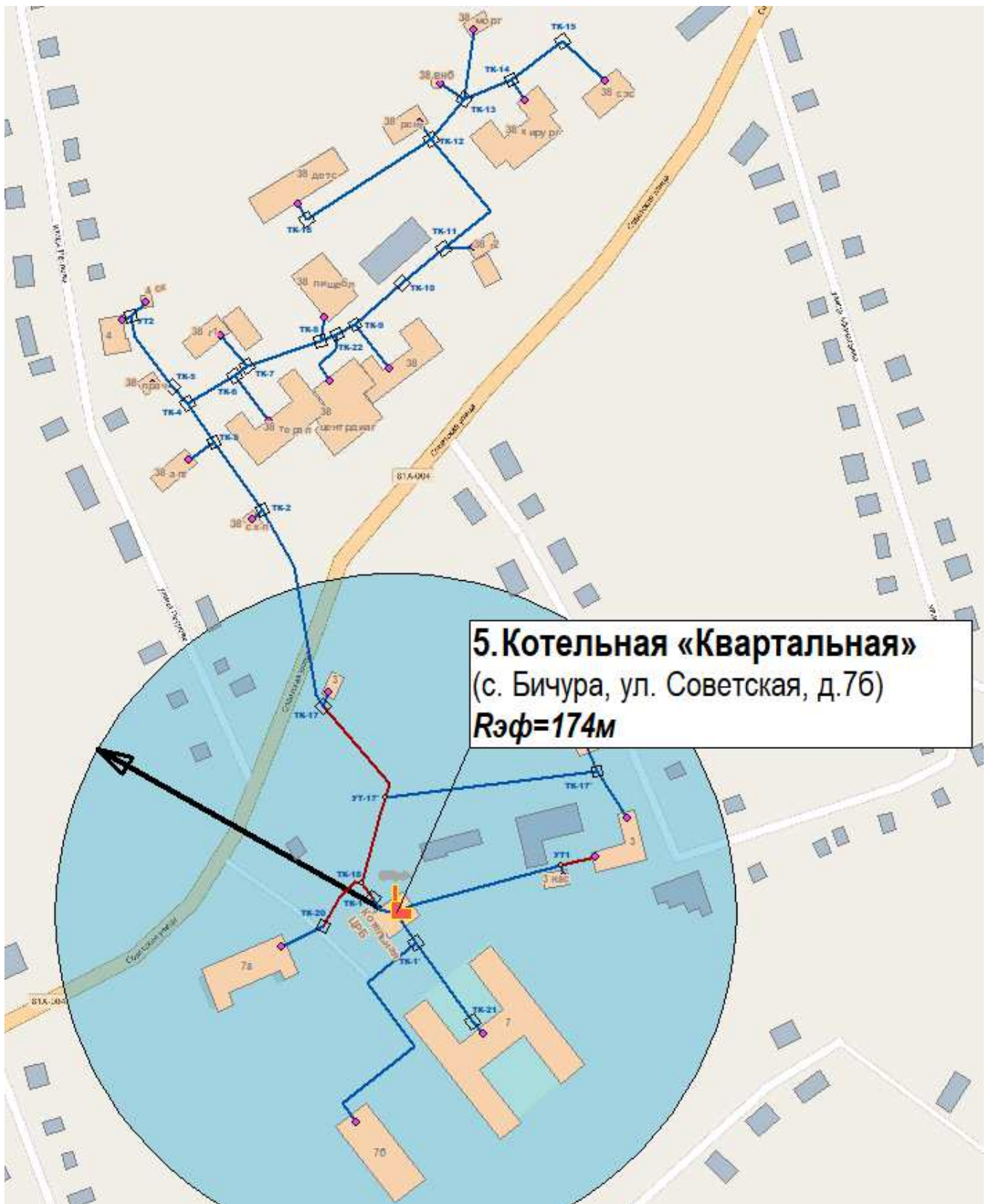
Рис. 2.61. Схема существующего радиуса эффективного теплоснабжения от котельной «Квартальная»
