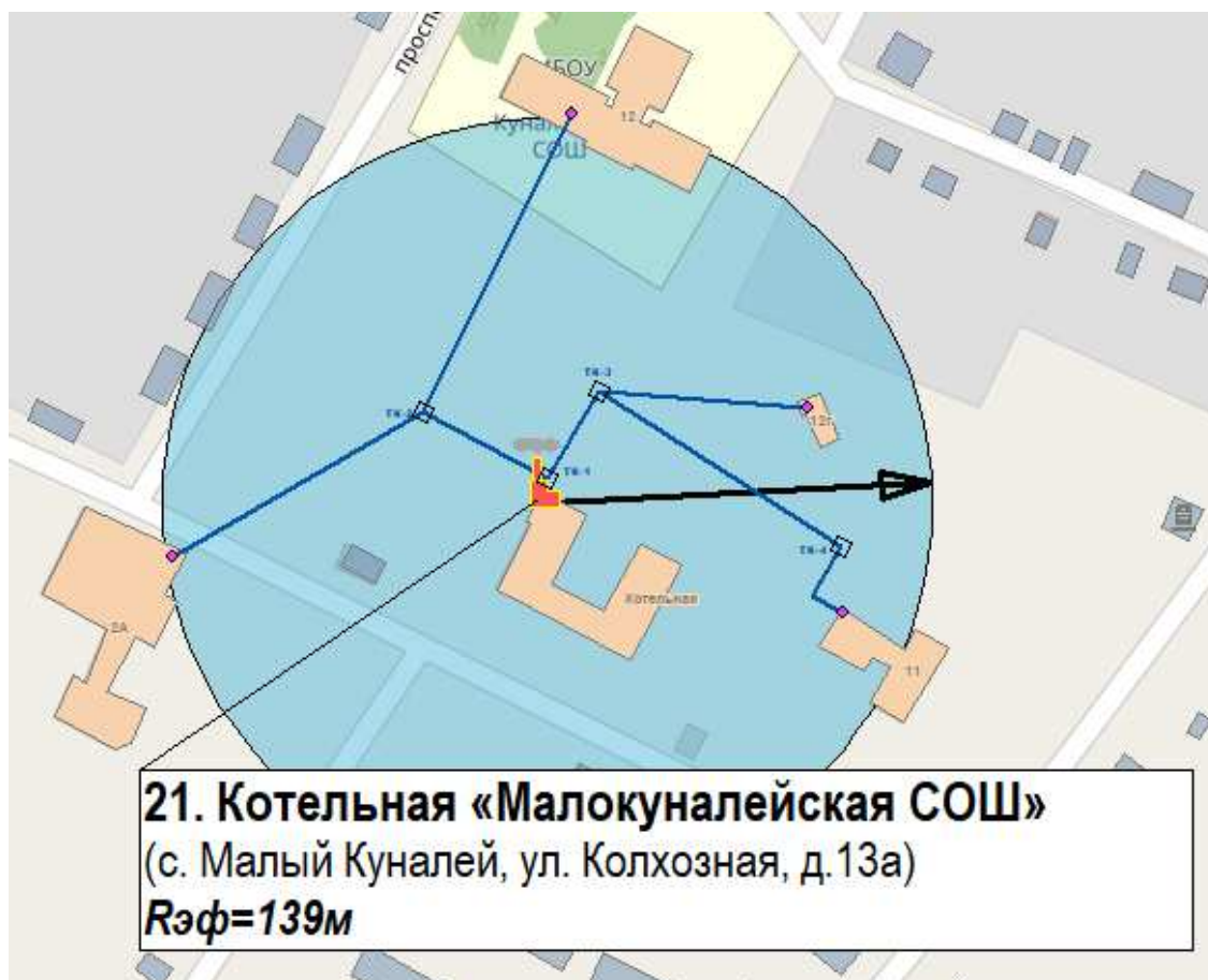
Рис. 2.77. Схема существующего радиуса эффективного теплоснабжения от котельной «Малокуналейская СОШ»
