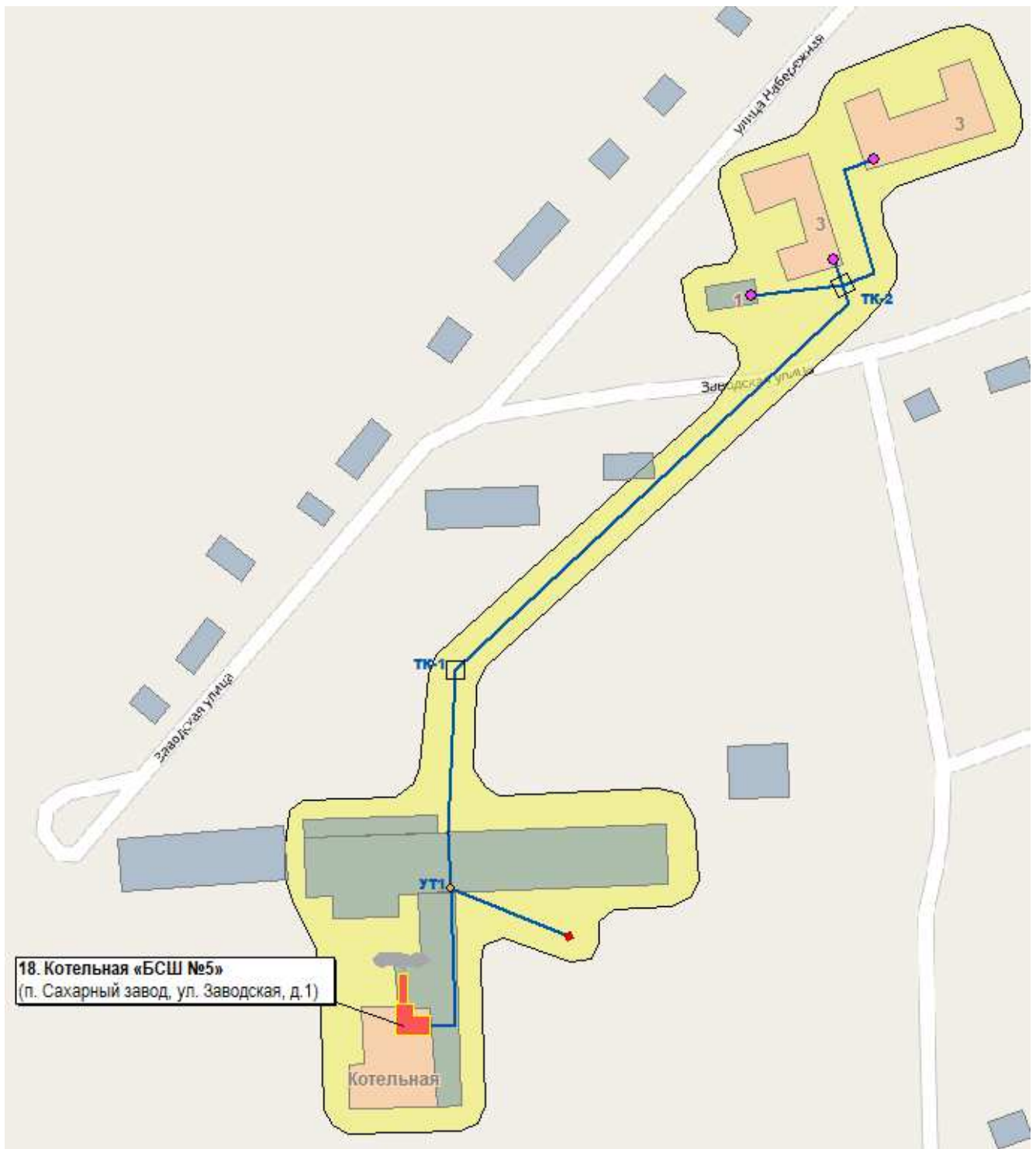
Рис. 2.18. Существующая зона действия системы теплоснабжения и централизованного источника тепловой энергии – котельной «БСШ №5»
