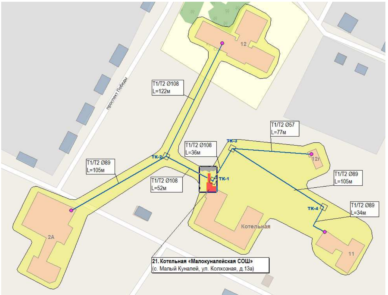
Рис. 2.49. Перспективная зона действия системы теплоснабжения и централизованного источника тепловой энергии – котельной «Малокуналейская СОШ»
