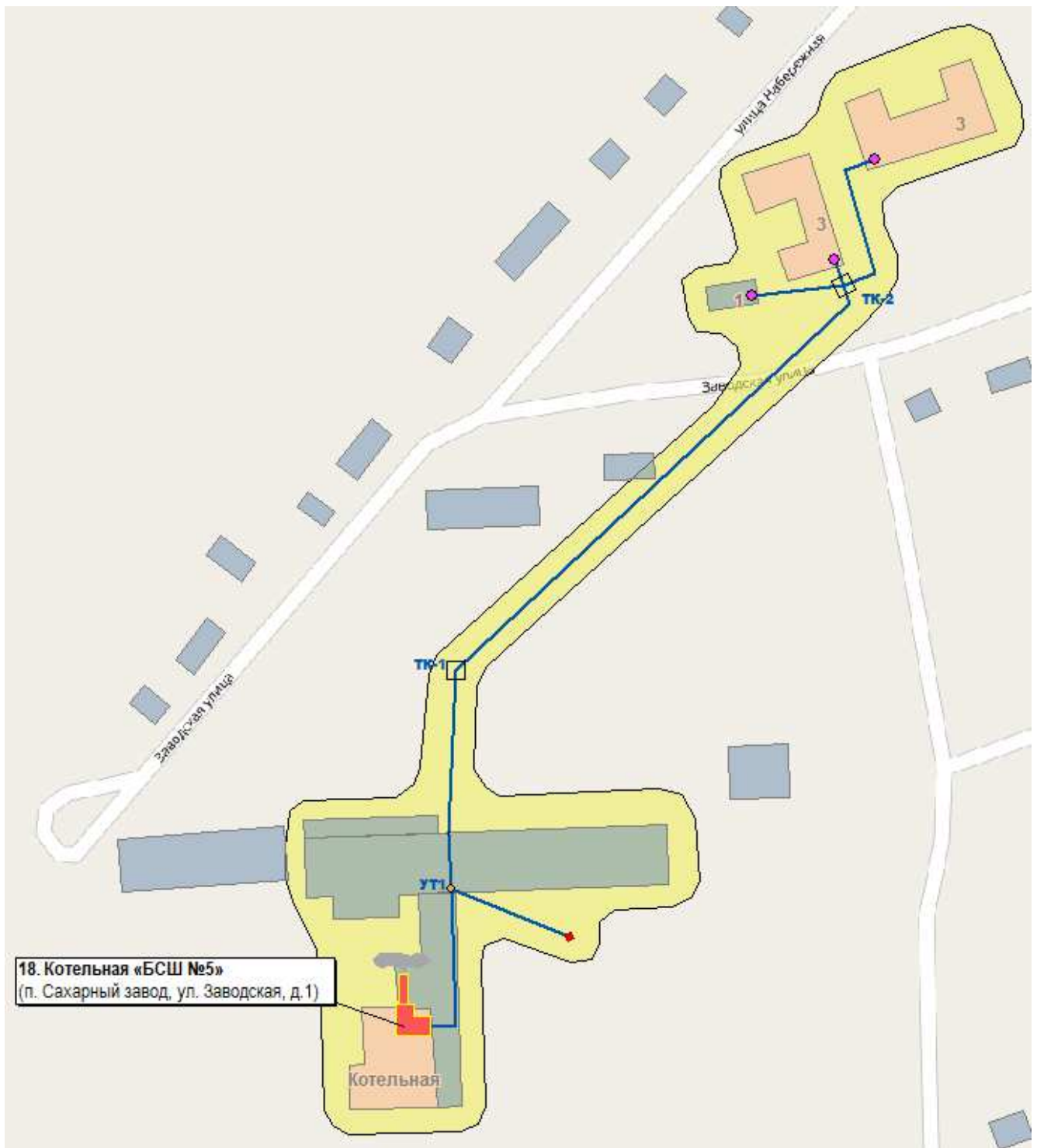
Рис. 2.46. Перспективная зона действия системы теплоснабжения и централизованного источника тепловой энергии – котельной «БСШ №5»
