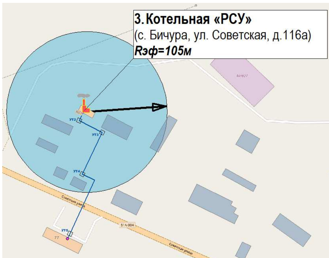
Рис. 2.59. Схема существующего радиуса эффективного теплоснабжения от котельной «PCУ»
