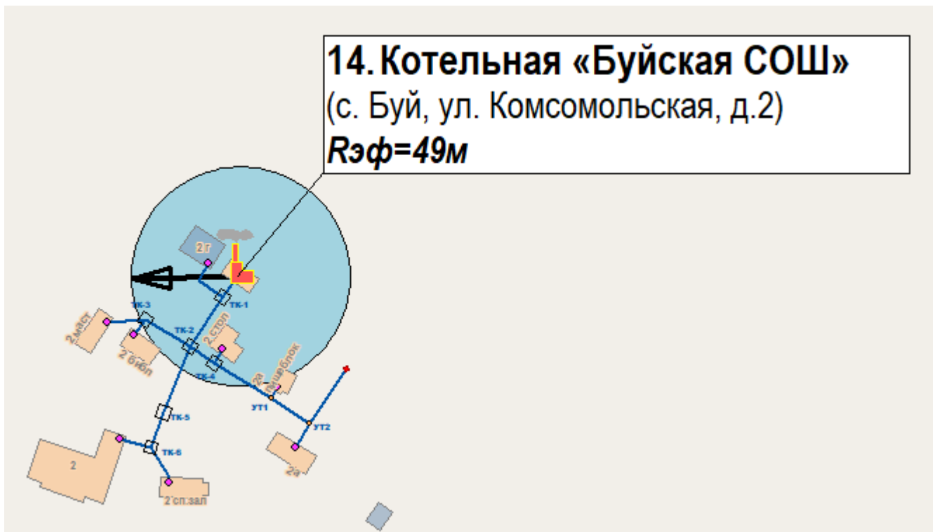
Рис. 2.70. Схема существующего радиуса эффективного теплоснабжения от котельной «Буйская СОШ»
