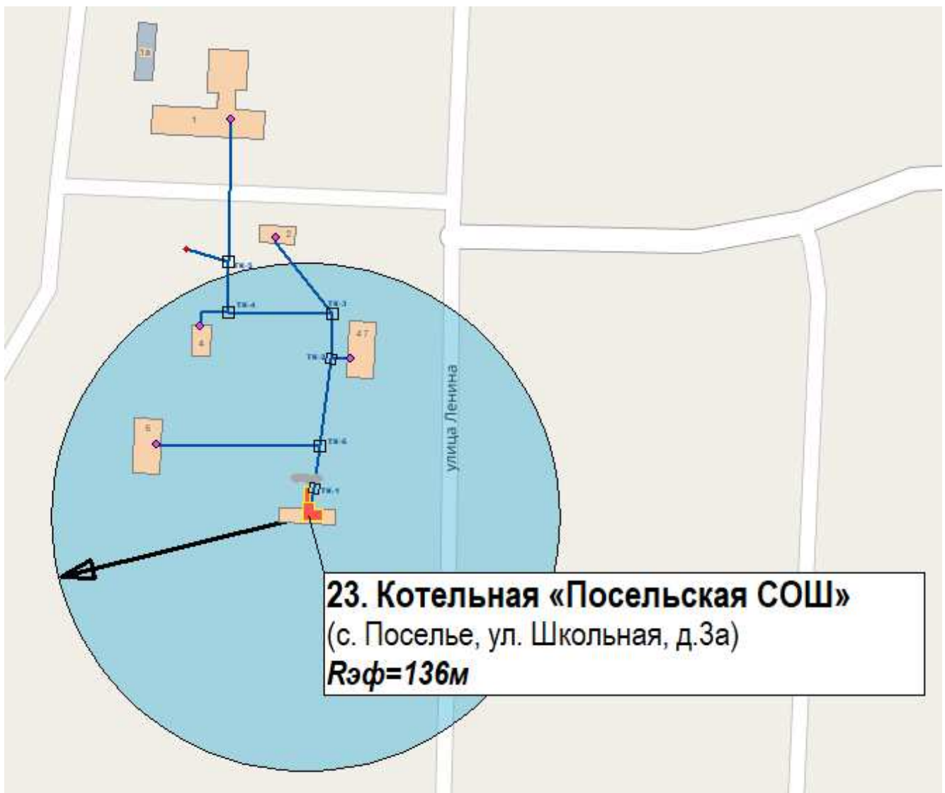
Рис. 2.79. Схема существующего радиуса эффективного теплоснабжения от котельной «Посельская СОШ»
