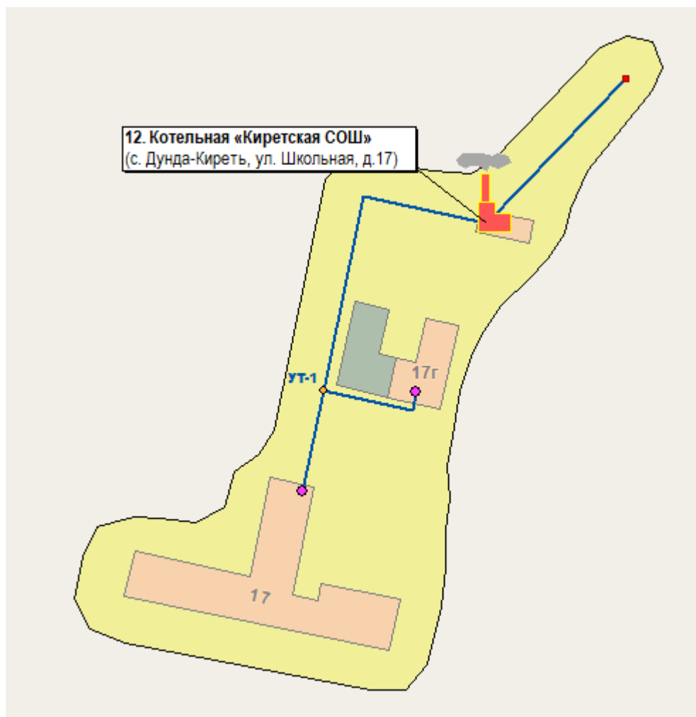
Рис. 2.40. Перспективная зона действия системы теплоснабжения и централизованного источника тепловой энергии – котельной «Киретская СОШ»
