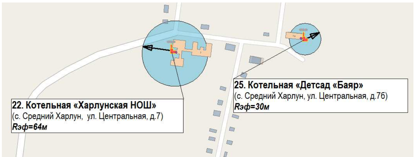
Рис. 2.78. Схема существующих радиусов эффективного теплоснабжения от котельной «Харлунская НОШ» и котельной «Детсад «Баяр»
