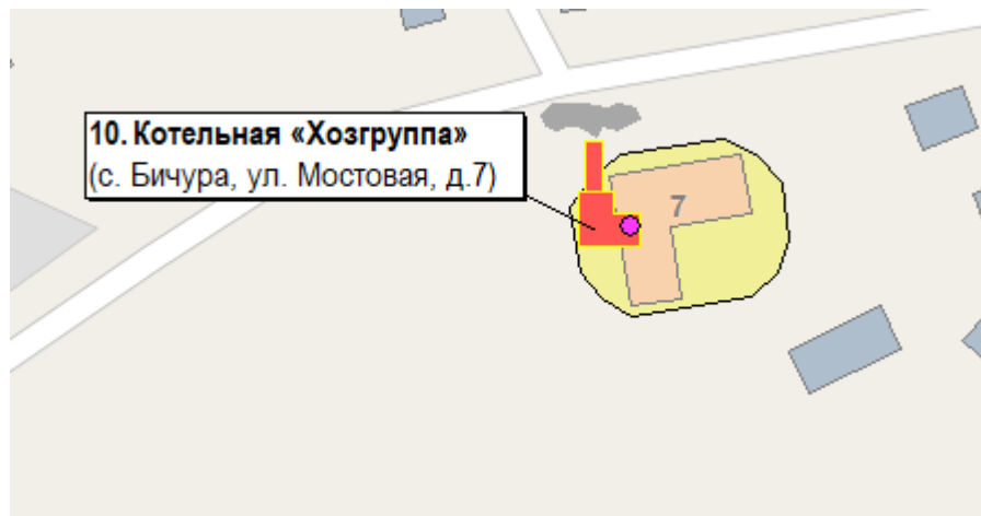
Рис. 2.10. Существующая зона действия системы теплоснабжения и централизованного источника тепловой энергии – котельной «Хозгруппа»
