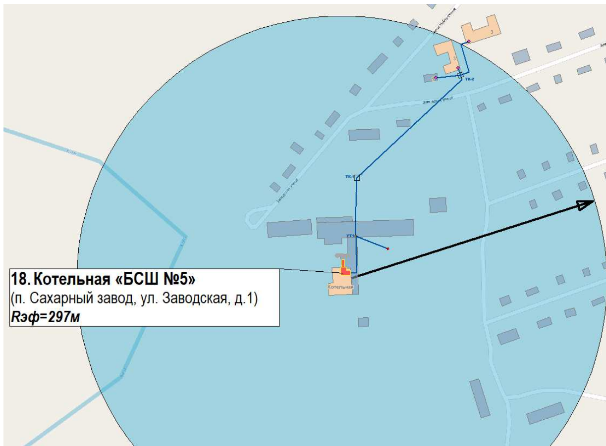
Рис. 2.74. Схема существующего радиуса эффективного теплоснабжения от котельной «БСШ №5»
