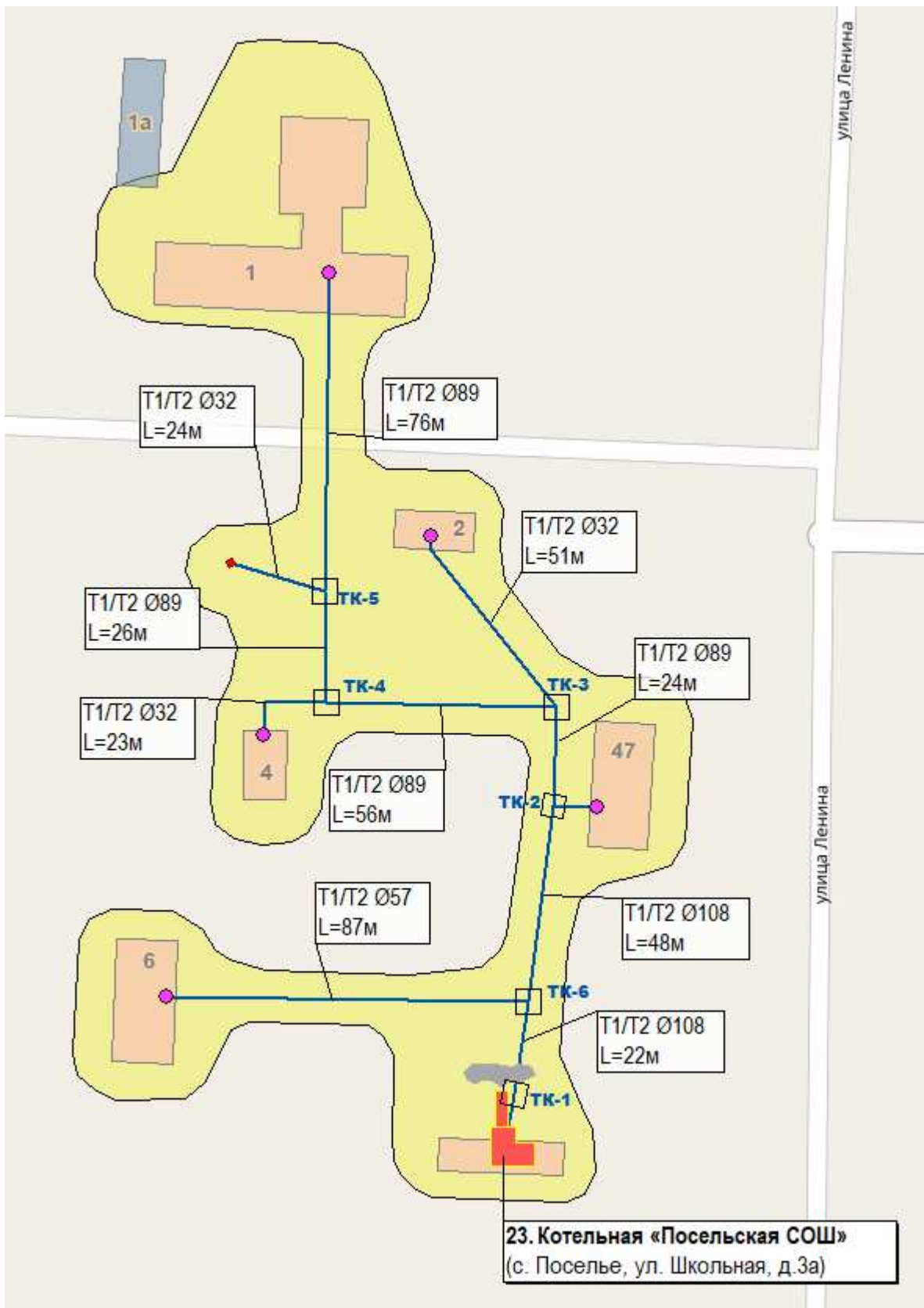
Рис. 2.51. Перспективная зона действия системы теплоснабжения и централизованного источника тепловой энергии – котельной «Посельская СОШ»
