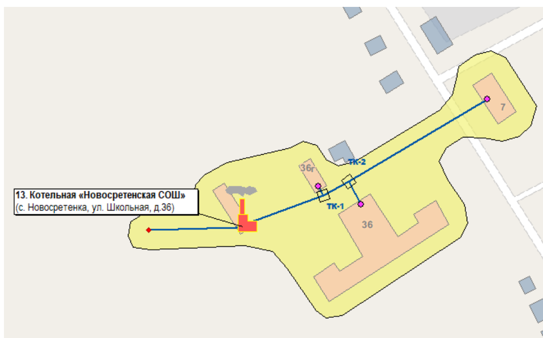
Рис. 2.41. Перспективная зона действия системы теплоснабжения и централизованного источника тепловой энергии – котельной «Новосретенская СОШ»
