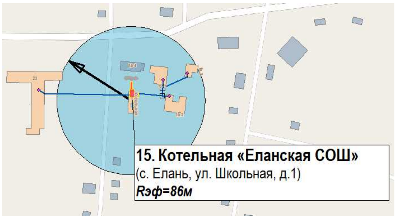
Рис. 2.71. Схема существующего радиуса эффективного теплоснабжения от котельной «Еланская СОШ»
